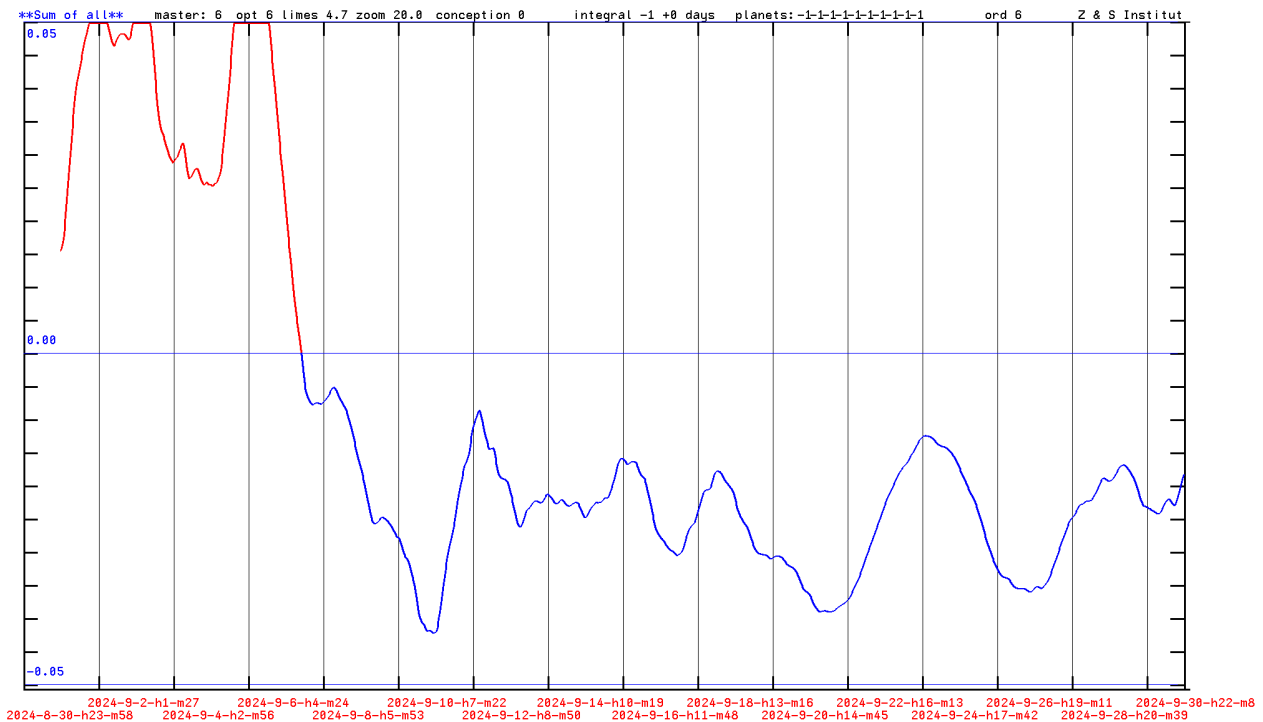
Abb. 7. Kurve des Musters A für den Zeitraum 2024-09. Oberhalb der Mittellinie ist die Wahrscheinlichkeit für ein Erdbeben des Musters A größer.
