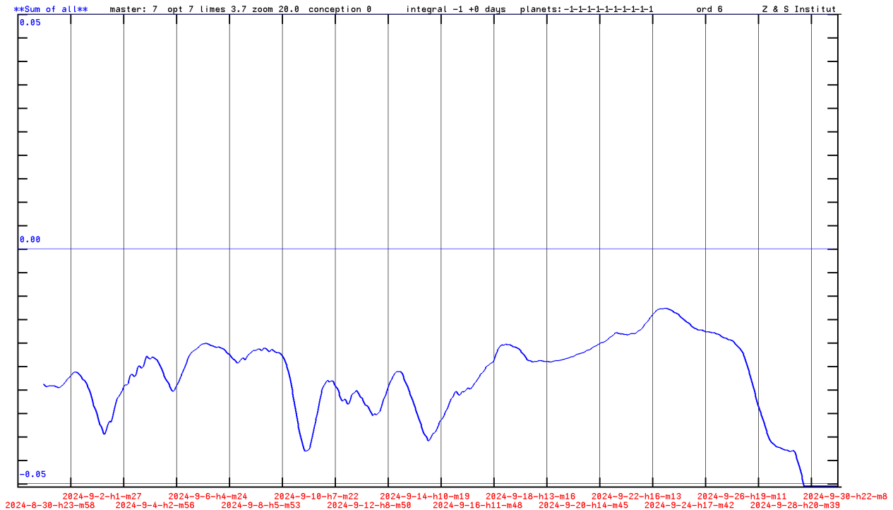
Abb. 8. Kurve des Musters B. 513-Erdbeben für den Zeitraum 2024-09. Oberhalb der Mittellinie ist die Wahrscheinlichkeit für ein Erdbeben des Musters A größer.
