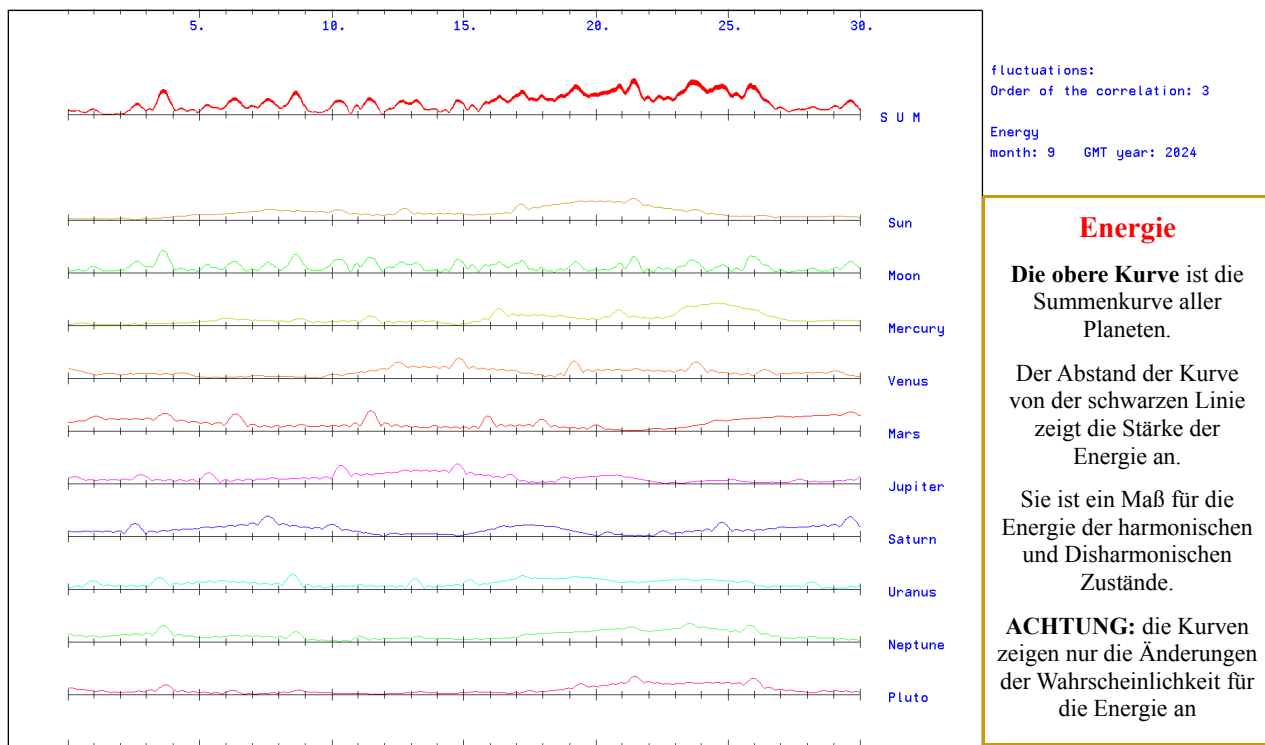
Abb. 3. Die Energie der Zeitqualität im September 2024
