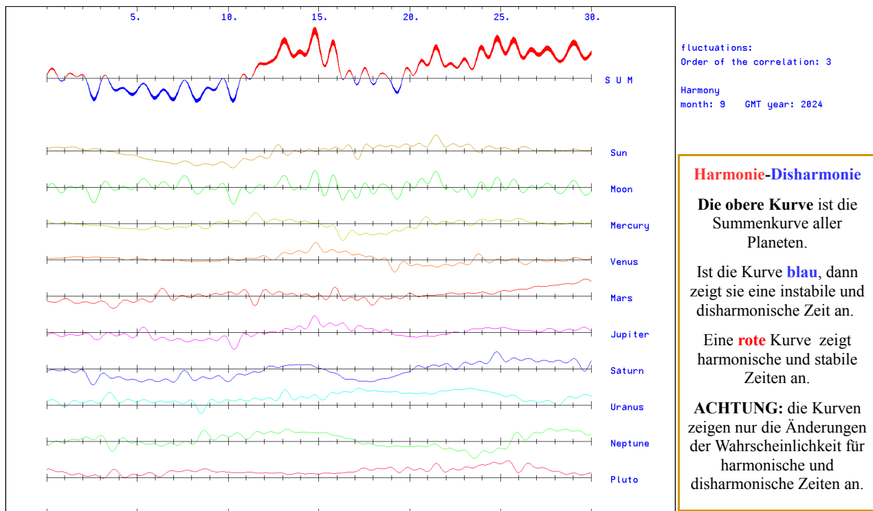
Abb. 1. Die Zeitqualität im September 2024; Vollmond ist am 18., Neumond am 3. September
